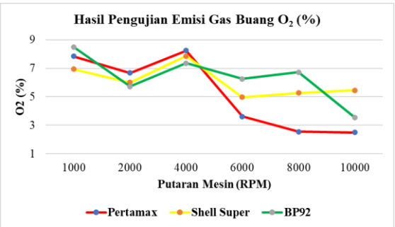
Gambar 8. Pengujian O 2 Emisi Gas Buang
