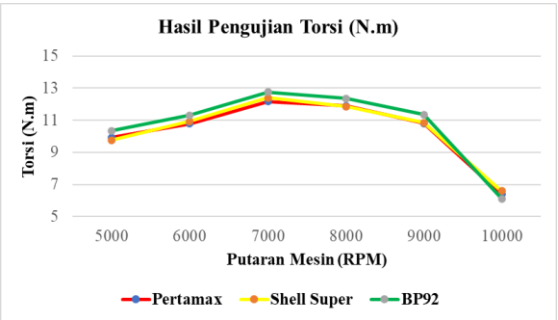
Gambar 4. Pengujian Torsi
