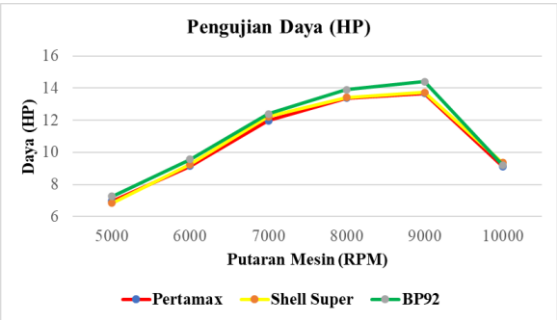
Gambar 3. Pengujian Daya
